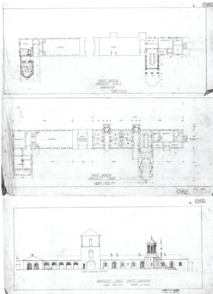
Fig.2 Proiectul de restaurare al Mănăstirii Snagov, arh. Ștefan Balș, 1943-1947 Sursa: I.N.P, https://www.stefan-bals.ro/cmi/Snagov.pdf consultat în data de 3 octombrie 2019
