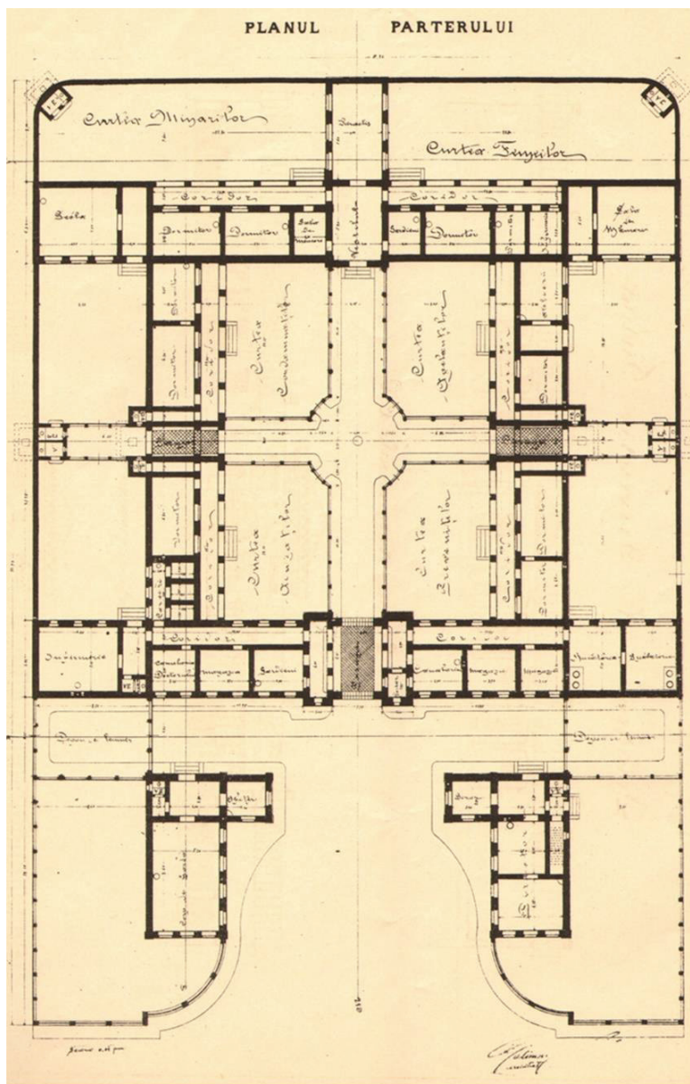
Fig.26 Penitenciarul Tulcea, plan, 1892 sursă: I.N. Socolescu (ed.), Analele arhitecturii și ale artelor cu care se leagă , anul III, 1892, nr.4
