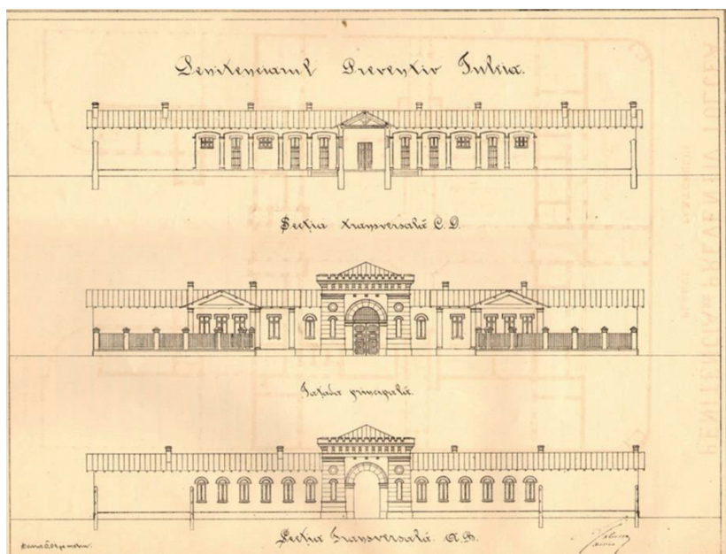
Fig.26 Penitenciarul Tulcea, fațade, 1892
