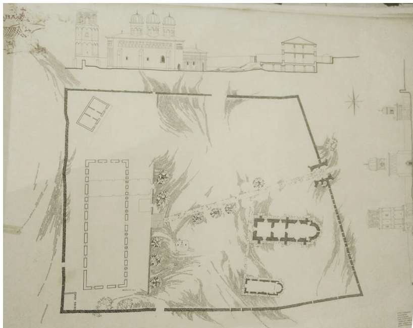
Fig.73 Planul Mănăstirii Dobrovăț, relevu, 1966 sursa: Arhiva Universității de Arhitectură și Urbanism „Ion Mincu” București, relevu nr. inv. R.108/96, planșa Plan de situație
