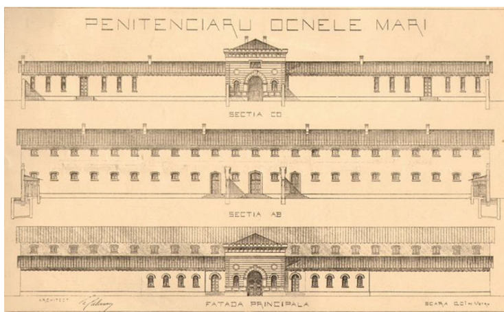
Fig.25. Penitenciarul Ocnele Mari, fațade, arh., Grigore Calinescu, 1891 sursa: I.N. Socolescu (ed.), Analele arhitecturii și ale artelor cu care se leagă , an II, 1891, nr.1-2
