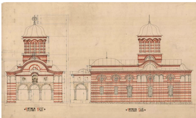
Fig.47 Mănăstirea Cozia, biserica, fațade și plan, relevu autor necunoscut, 1958 sursa: Arhiva Universității de Arhitectură și Urbanism „Ion Mincu” București, Relevu Rv.146, planșa Rv.146.03 Biserica Sf. Treime: Fațadă vest, Fațadă sud, https://relevee.uauim.ro/m104
