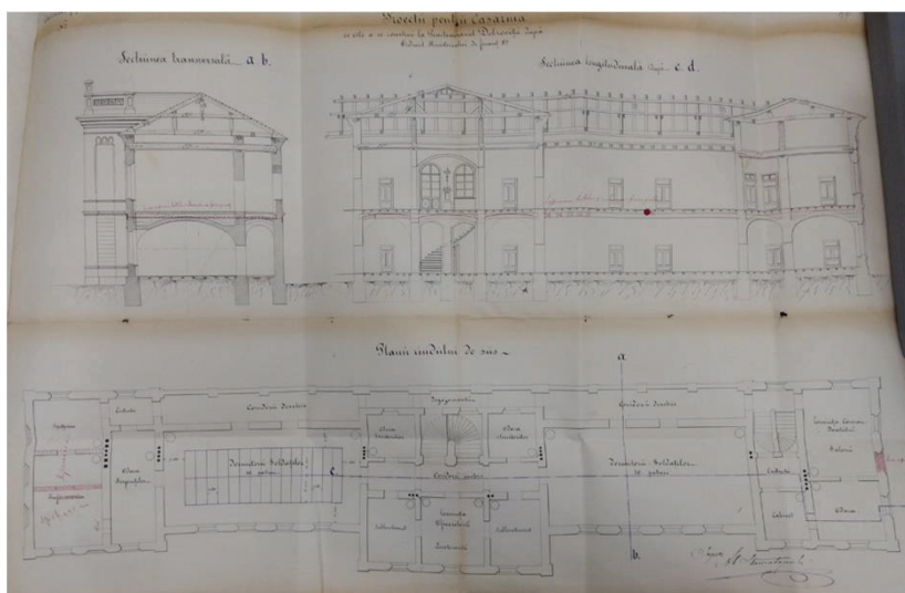
Fig. 63 Cazarma Dobrovăț, varianta II, plan etaj și secțiune, 1871 sursa: A.N.I.C. fond Direcția Generală a Penitenciarelor, dosar 2/1870, f. 75
