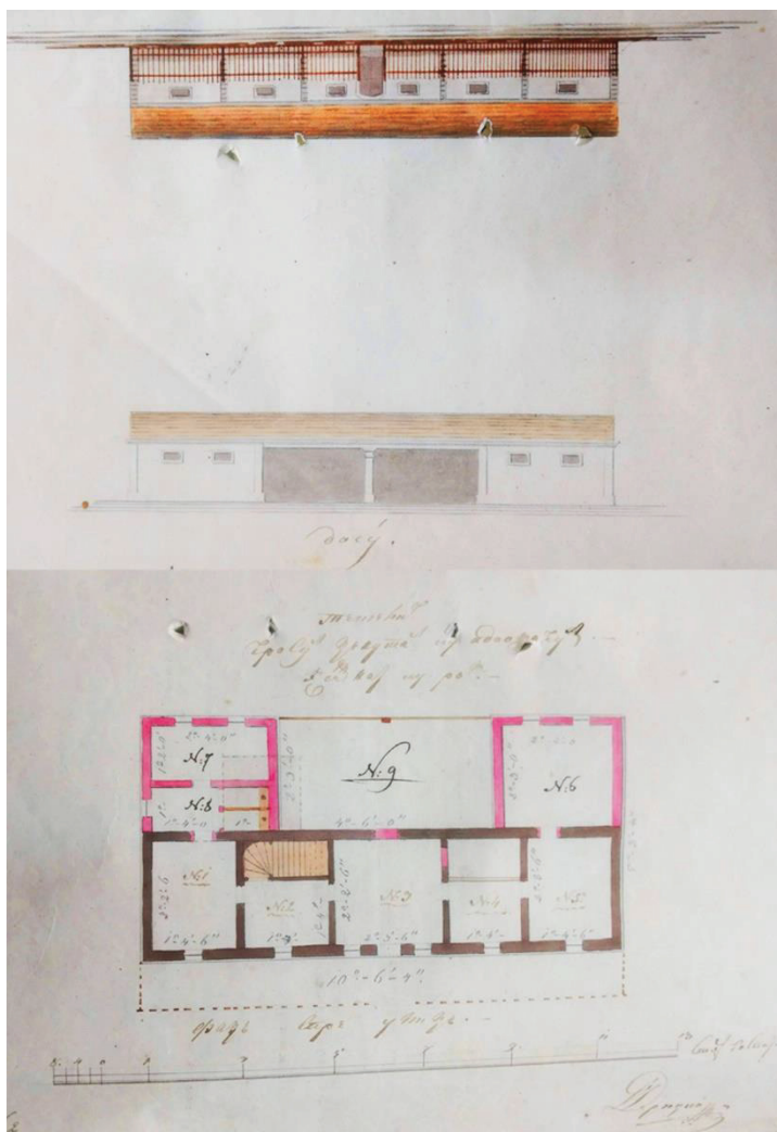
Fig.14 Arest din Moldova, varianta III, 1849 sursa: A.N.R. Iași fond M.L.P., dosar 429/1849, fila 82
