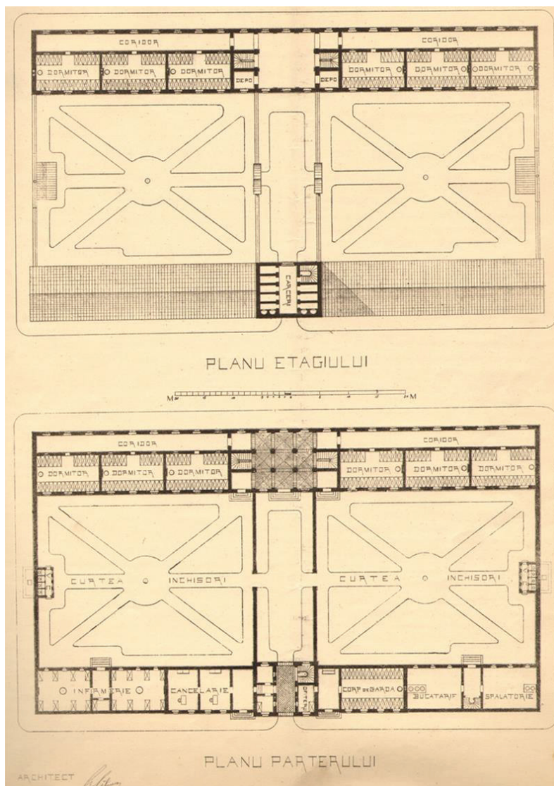
Fig.24. Penitenciarul Ocele Mari, planuri, arh., Grigore Calinescu, 1891 sursa: I.N. Socolescu (ed.), Analele arhitecturii și ale artelor cu care se leagă , an II, 1891, nr.1-2
