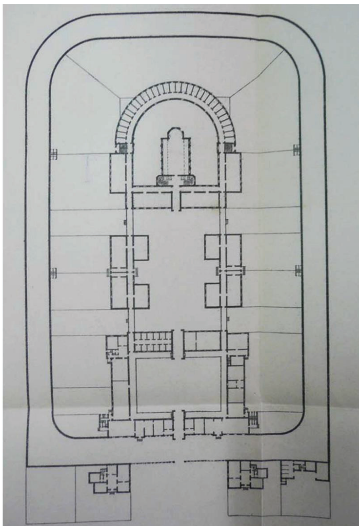
Fig.31 Planul tip al penitenciarelor din Craiova și Galați, 1890-1900 sursa: Grigore I. Dianu, Închisorilor din Romania, studiu comparativ, legi si obiceiri , Tipografia Curții Regale G. Göbel și fii, București, 1901, pl. VL
