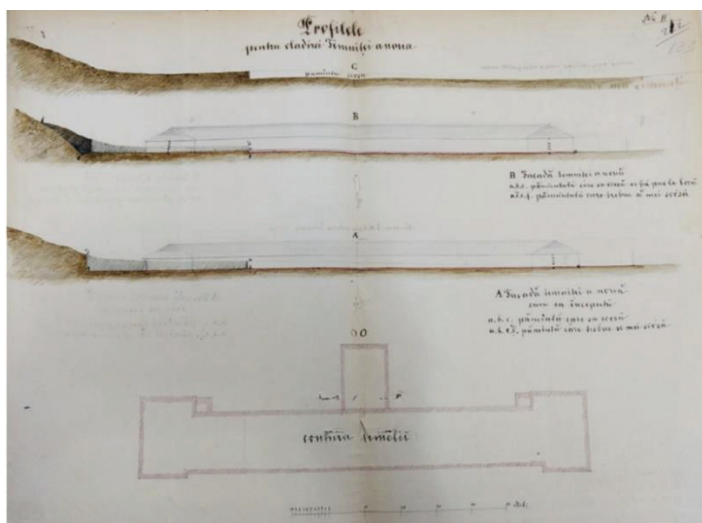
Fig.21 Profile, închisoarea Ocnele Mari, 1868 sursa: A.N.I.C. fond Vornicia Temnițelor, dosar 2/1868, fila 123
