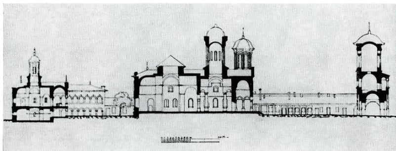
Fig.85 Secțiune longitudinală a primei incinte a Mănăstirii Văcărești, după N. Ghica Budești, Evoluția arhitecturii în Muntenia și Oltenia, sec. al XVIII-lea , pl. CCCLXIV
