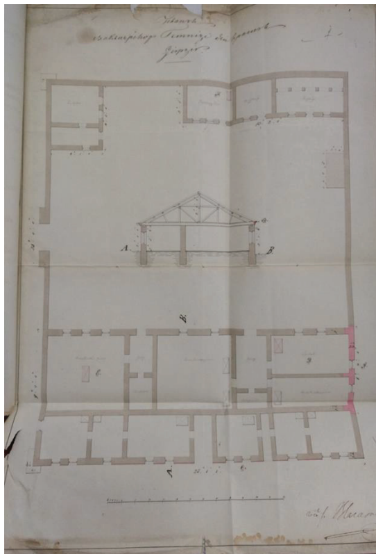
Fig.19 Temnița Giurgiu, Vladimir von Blaremborg, 1844 sursa: A.N.I.C. fond M.L.P. dosar 57/1844, fila 7
