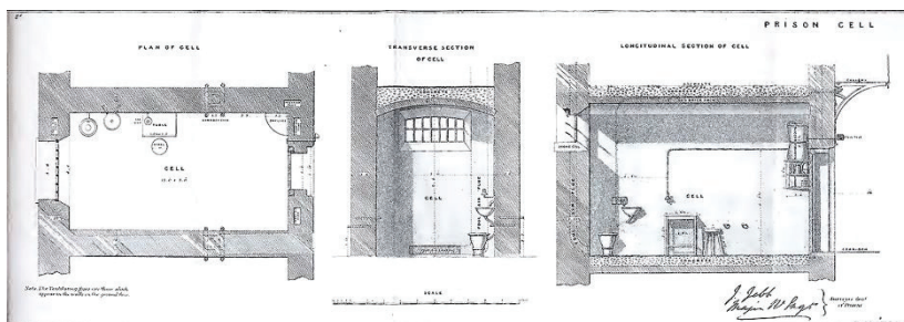
Fig. 52 Celulă din închisoarea Pentonville, Londra, 1844
