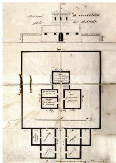
Fig.10 Maison de correction pour les districts , Vladimir von Blaremborg, 1833 sursa: A.N.I.C. fond Vornicia temnițelor, dosar 26/1833, fila 9
