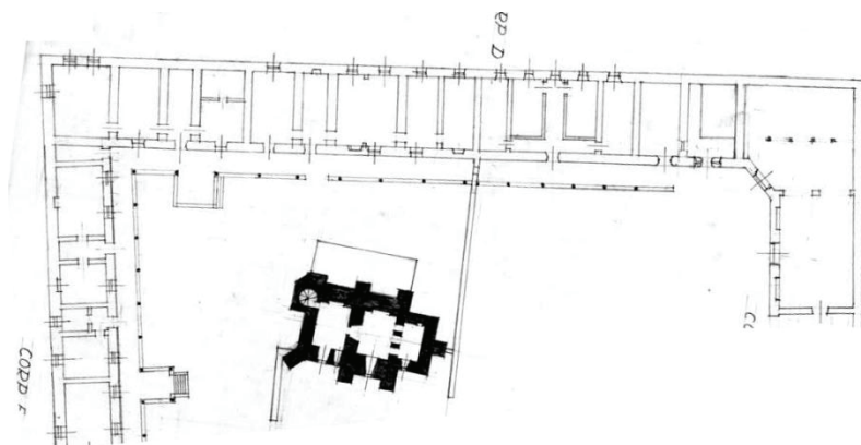
Fig.55 Mănăstirea Pângărați, patru incinte, relevu arh. Stefan Balș, 1943 sursa: Arhiva Institutului Național al Patrimoniului, fond Comisia Monumentelor Istorice, jud. Neamț, loc. Pângărați https://stefan-bals.ro/cmi/Manastirea-Pangarati.pdf consultata la data de 3 octombrie 2019
