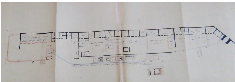
Fig.16 Temnița Capitalei , arh. Alexander von Montbach, 1853 sursa: A.N.I.C. fond M.L.P. dosar 94/1859
