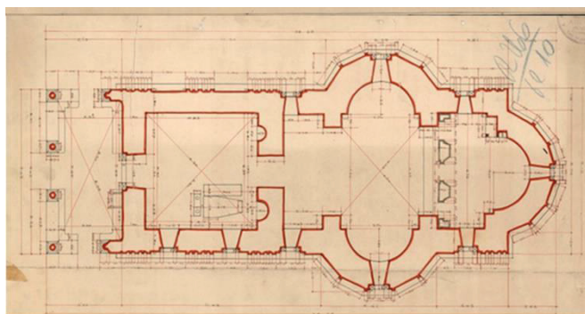
Fig.48 Mănăstirea Cozia, biserica, fațade și plan, relevu, autor necunoscut 1958 sursa: Arhiva Universității de Arhitectură și Urbanism „Ion Mincu” București, Relevu Rv.146, planșa Rv.146.04 Biserica Sf. Treime: Plan https://relevee.uauim.ro/m104
