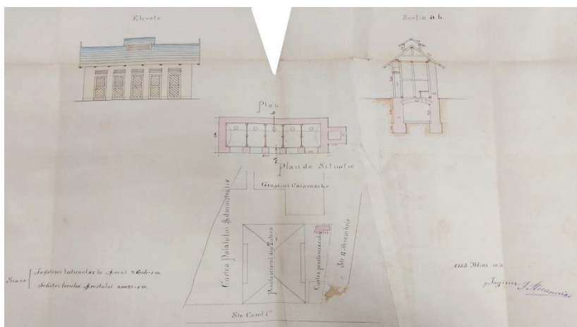
Fig.65 Proiect toaleta pentru penitenciarul Tulcea, ing. I. Stoianovici, 1886 Sursa: A.N.I.C., fond Vornicia Temnițelor, dosar 1/1885
