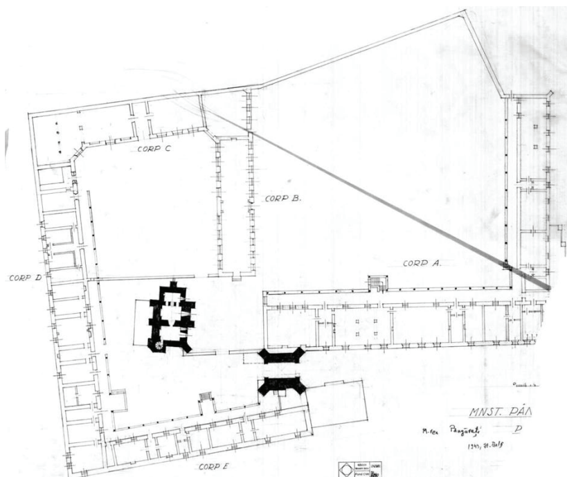
Fig.46 Mănăstirea Pângărați, patru incinte, relevu arh. Stefan Balș, 1943 sursa: Arhiva INP, fond Comisia Monumentelor Istorice, jud. Neamț, loc. Pângărați https://stefan-bals.ro/cmi/Manastirea-Pangarati.pdf consultata la data de 3 octombrie 2019
