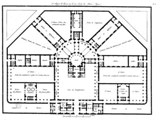
Fig.34 Proiect pentru închisoare, Paris sursă: Luis Pierre Baltard, Architectonographie de Prisons , 1929, pl.XII
