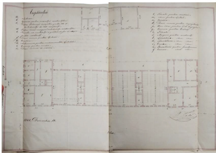
Fig.23 Plan de situație închisoarea Ocna Slănic, 1860 sursa: A.N.I.C. fond Vornicia Temnițelor, dosar 127/1860
