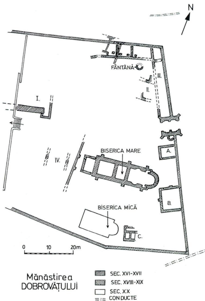
Fig.75 Plan de situație cu marcarea vestigiilor medievale și mai târzii, etape de construcție, autori V.M. Pușcașu și N.N. Pușcașu sursa: V.M. Pușcașu și N.N. Pușcașu, Mănăstirea Dobrovățului: monografie arheologică și istorică , Editura Mitropolit Iacov Putneanul, 2012, planșa 24
