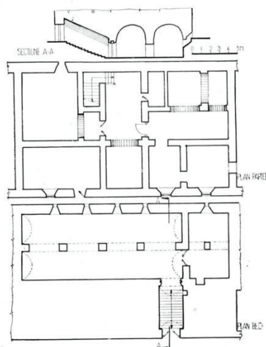
Fig.82 Beciul arhondaricului fostei Mănăstiri Mislea sursa: Cătălin Hoinărescu, „Ctitorii cantacuziene din Prahova” în RMM_MIA , nr.1, 1985, fig.3
