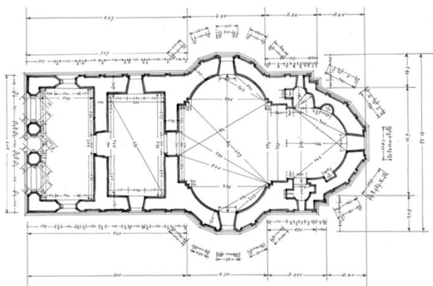
Fig. 49 Mănăstirea Plătărești, biserica plan și secțiuni, relevu 1936, autor Aurora Gabrielescu
